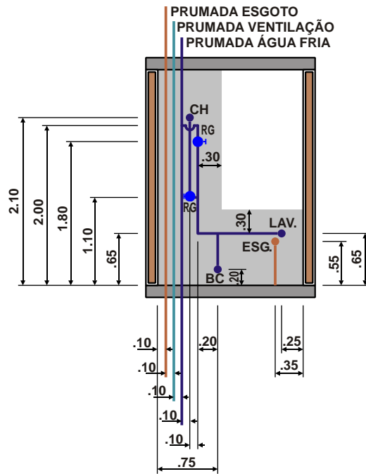
VISTA 1 WC EMPREGADA
